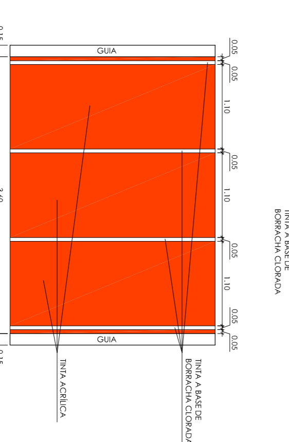
DETALHE - PISTA DE CORRIDA ESC 1/50
